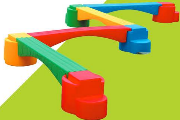
型号 LE.MQ.001 尺寸 4200*1760*290 mm 材质 LLDPE 体积 0.5m 3
