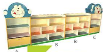
型号 LE.SJ.032 尺寸 A.650*300*1300 B.1200*300*900 C.650*300*1300 mm 材质 LLDPE 体积 0.8m 3
